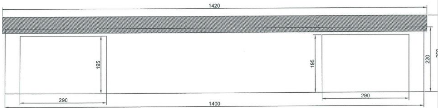
Rzut garażu 14x5 Ściana tylna
